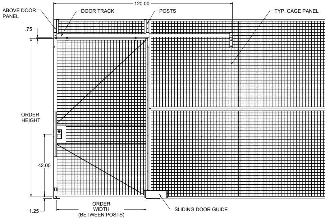
Dimensions
